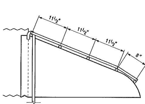
LONGITUDINAL VIEW
