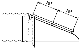
LONGITUDINAL VIEW
