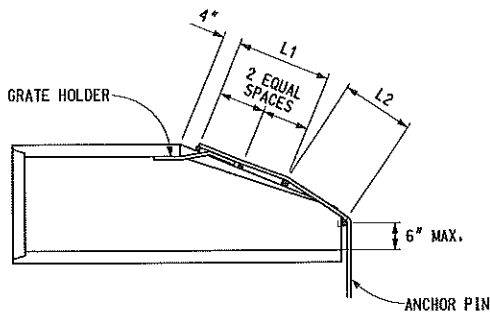
LONGITUDINAL SECTION
