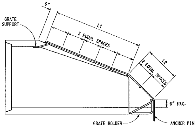
LONGITUDINAL SECTION
